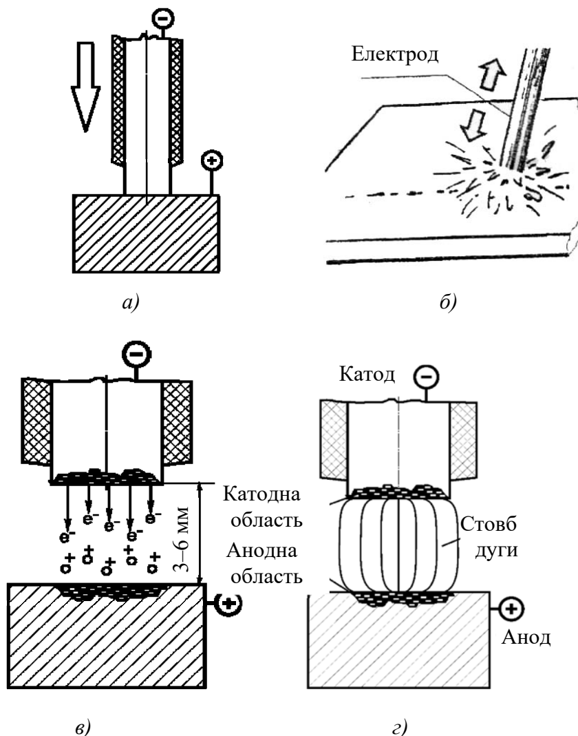
Рисунок 9.1 – Запалювання електричної дуги: а) – коротке замикання; б) – з) – етапи формування стабільної дуги
