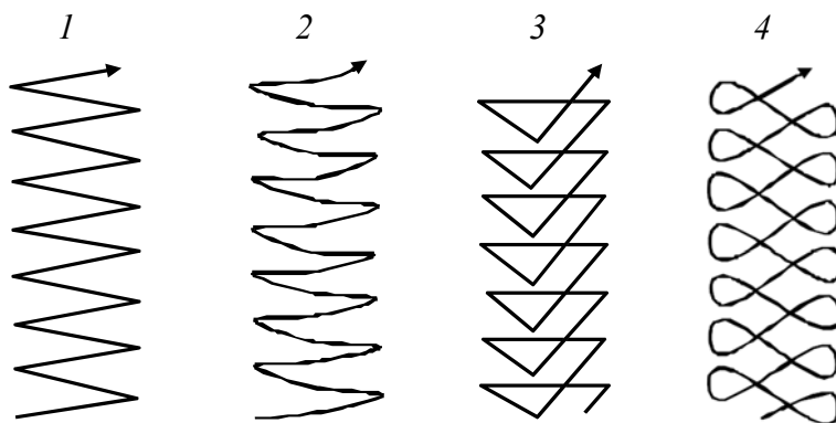
Рисунок 9.4 – Види поперечних переміщень кінця електрода:
