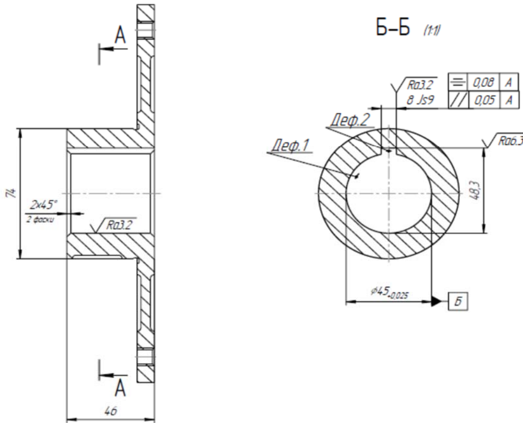
Рисунок 11.1 – Ескіз ремонтного кресленика деталі
