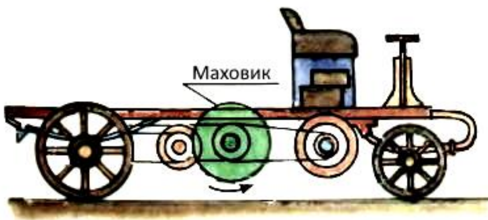
Рисунок 4.26 – Концептуальна схема та принцип дії жиробуса
