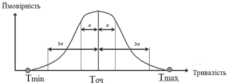
Рис. 2.16. Графік щільності розподілу ймовірності загальної тривалості проекту
