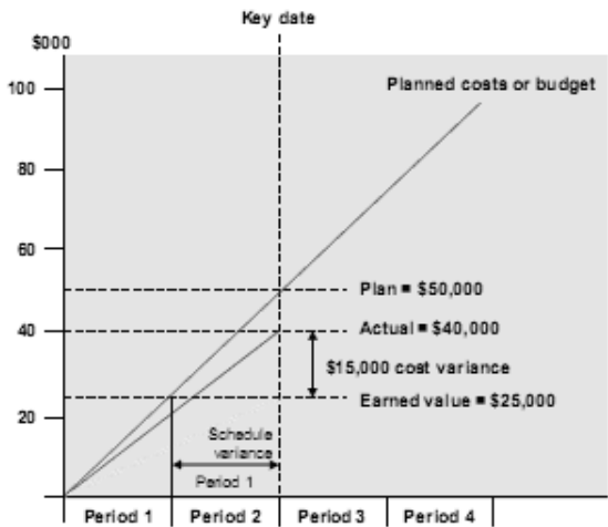
Рис. 2.24. Графік виміру EV на контрольну дату
