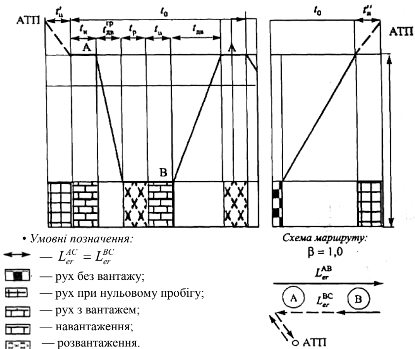
Рис. 5.5. Графік роботи автомобіля на маятниковому маршруті з неповністю навантаженим пробігом
