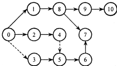
Рис. 5.2. Сітьовий графік
