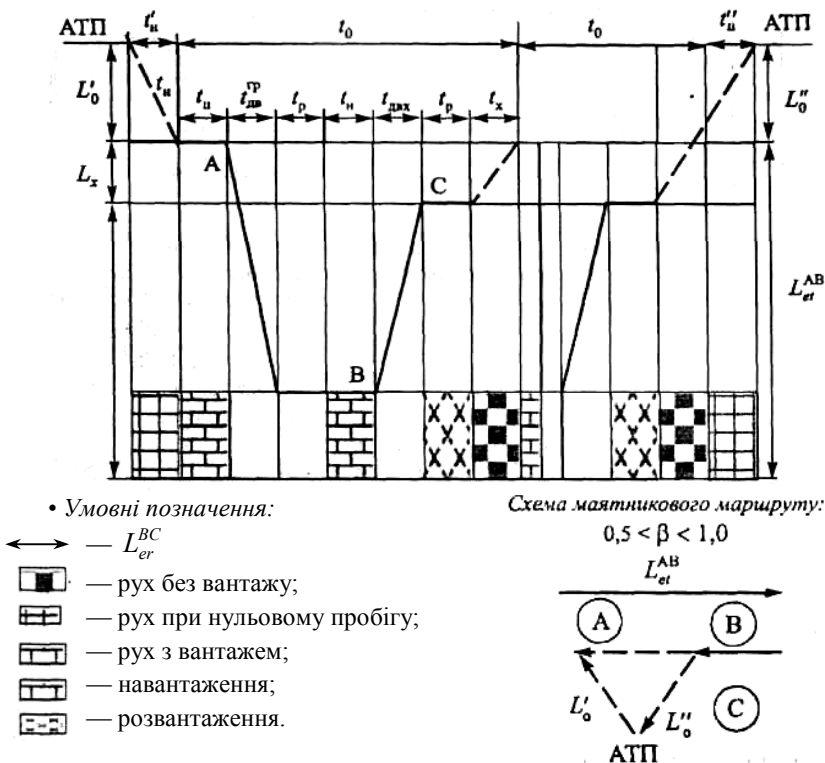
Рис. 5.4. Графік роботи автомобіля на маятниковому маршруті з неповністю навантаженим пробігом
